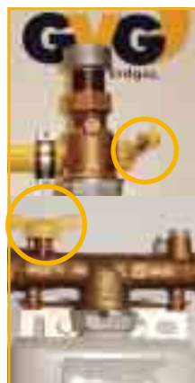
Oben: Zwei gängige Modelle des Hahns am Zähler. Hier kann die Gaszufuhr gestoppt werden
